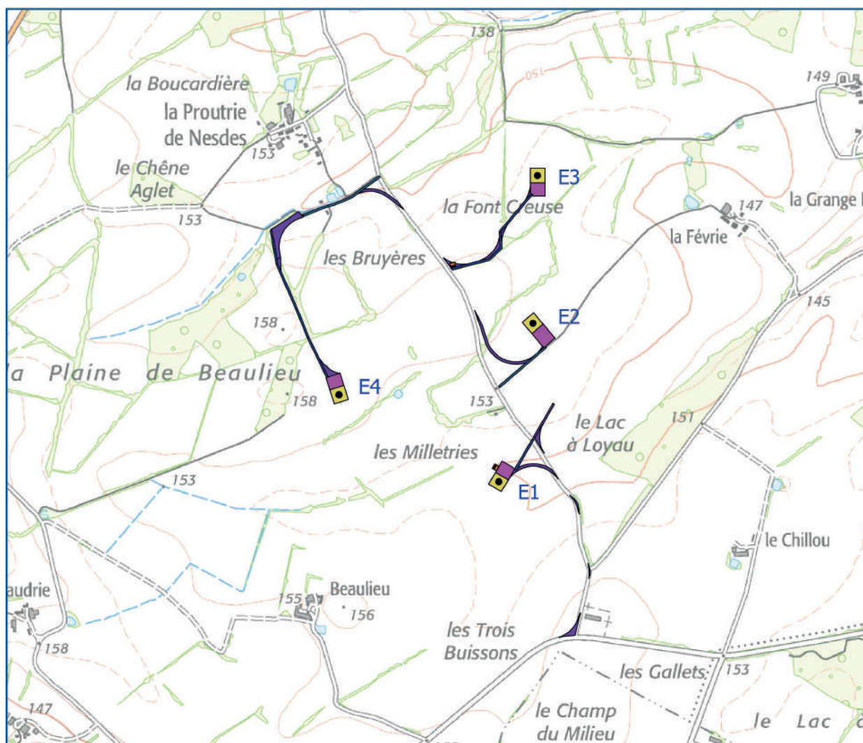
Parc éolien de La Plaine de Beaulieu – Implantation finale
